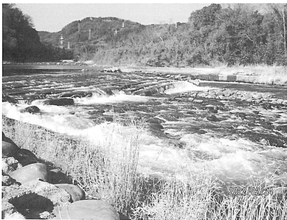
初瀬新井手の取り入れ口せき（場所：向原 うず河原）
